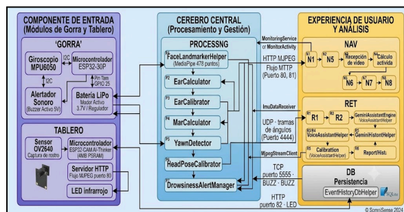
Fig. 8. Arquitectura de clases y flujo de datos del aplicativo móvil SomniSense (versión
