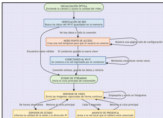
Fig. 6. Máquina de estados finitos del nodo central del tablero.
