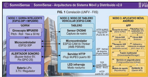
Fig. 1. Diagrama de bloques del sistema distribuido de alerta de fatiga: organización de los nodos portátil, central y de procesamiento móvil, módulos de reporte e inteligencia artificial, interfaces de comunicación inalámbrica y periféricos de salida física.
